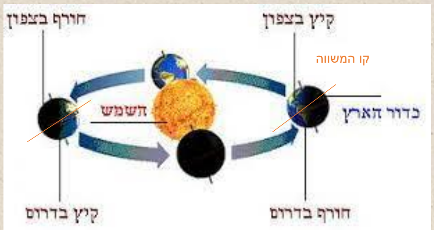
נטיית כדור הארץ והעונות.
